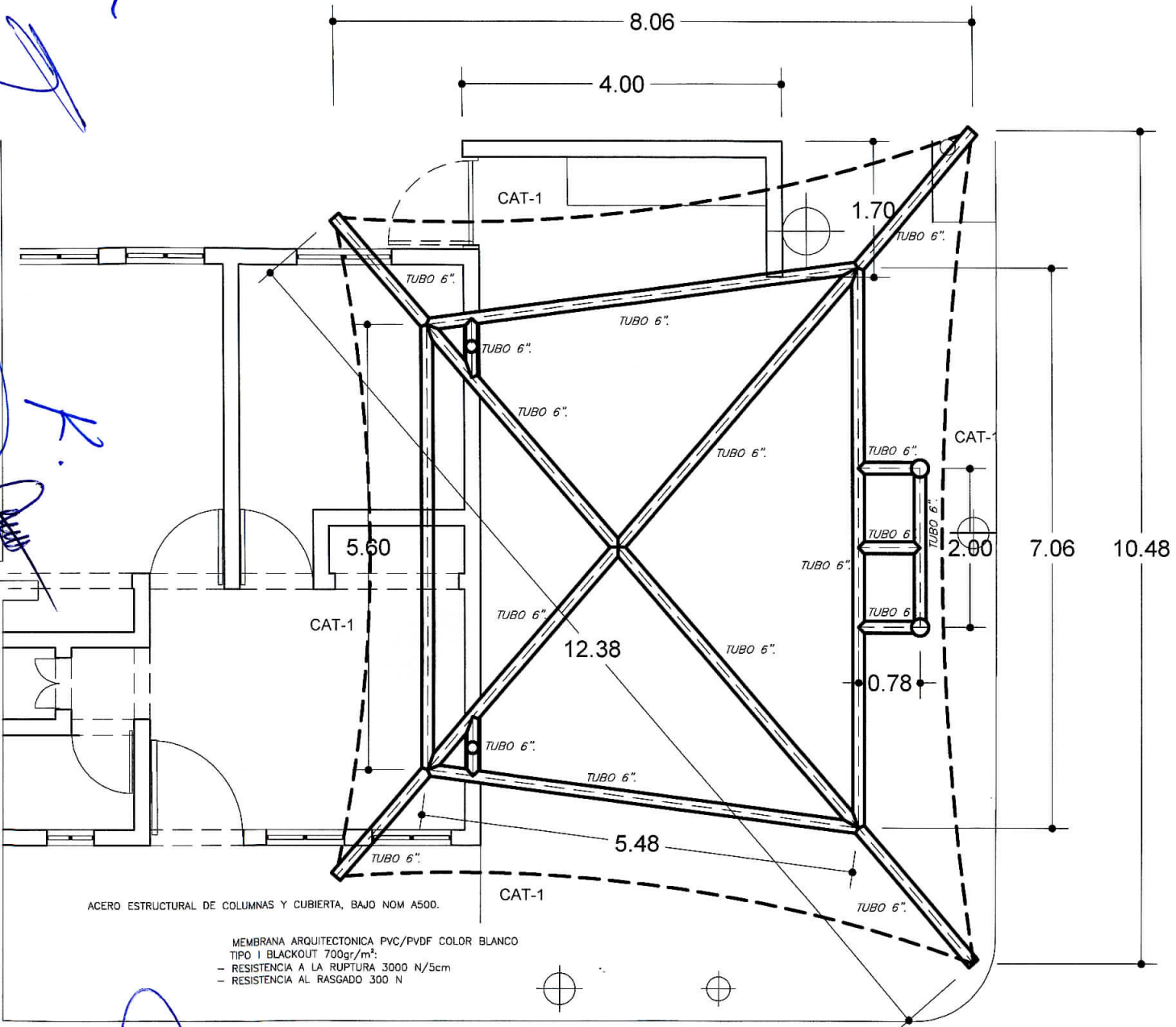
PLANTA DE ESTRUCTURACION DE CUBIERTA TALLER. ESC. 1:20
