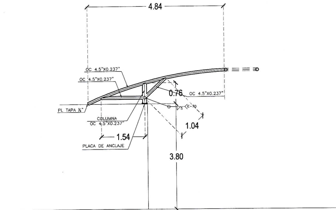
SECCION VIGA V-2
