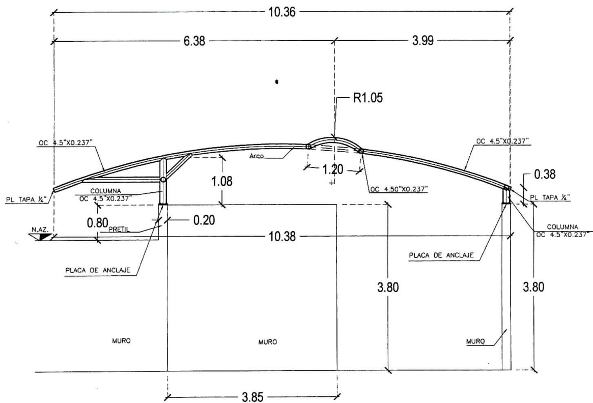
SECCION MARCO MA-1
