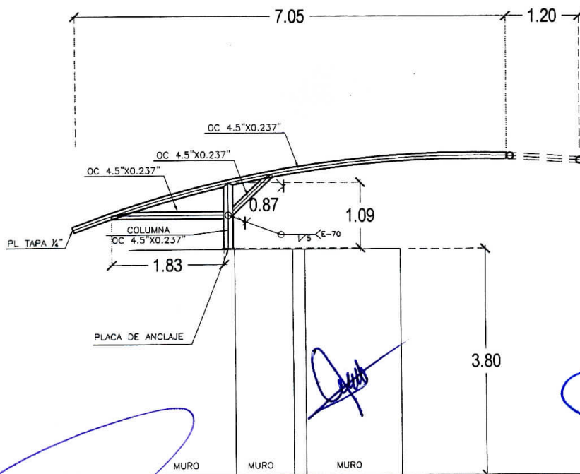
SECCION VIGA V-1
