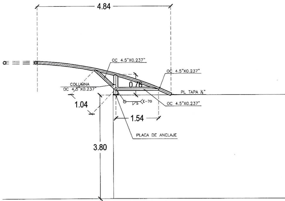
SECCION VIGA V-5
