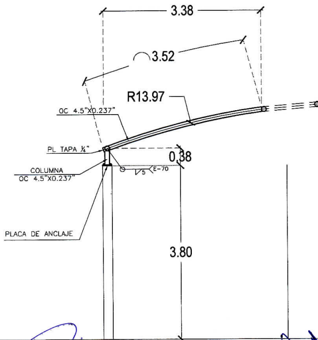
SECCION VIGA V-3
