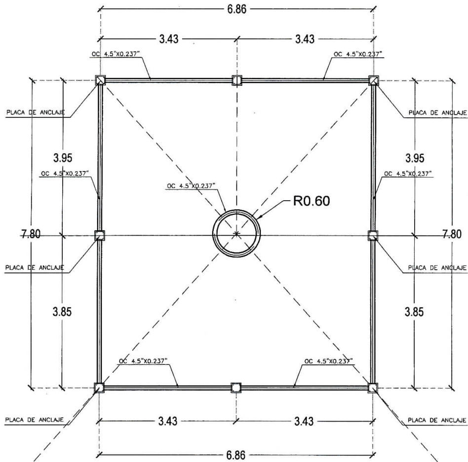
MARCO ESTRUCTURAL
