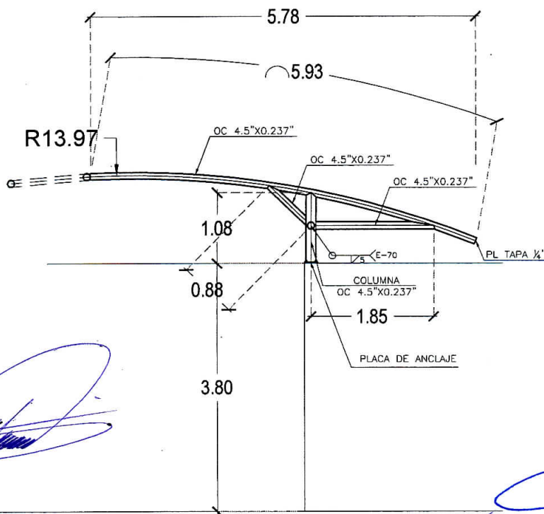
SECCION VIGA V-6
