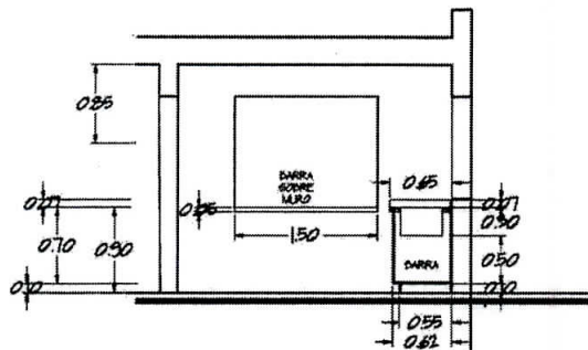
VISTA SECCION DE COCINA INTEGRADA
