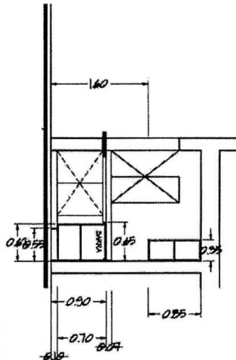
VISTA SECCION DE COCINA INTEGRADA
