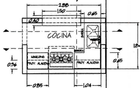
VISTA SECCION DE COCINA INTEGRADA
