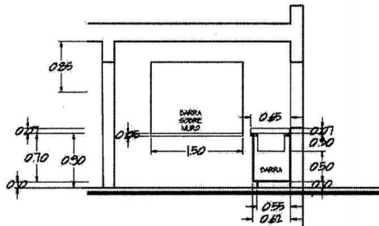
VISTA SECCION DE COCINA INTEGRADA
