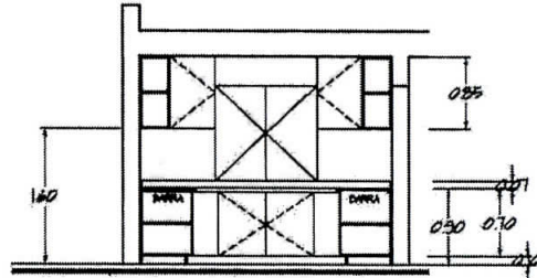
VISTA SECCION DE COCINA INTEGRADA
